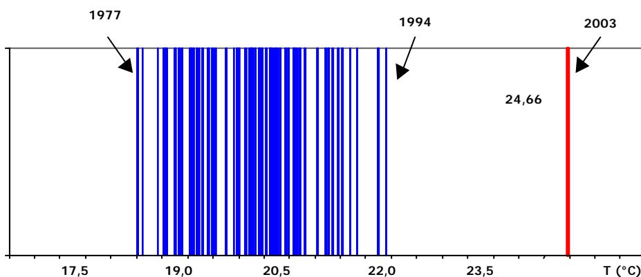
Grafico 1: Distribuzione delle temperature medie (media delle medie giornaliere) estive a Locarno-Monti, 1935-2003. (Fonte: MeteoSvizzera).
