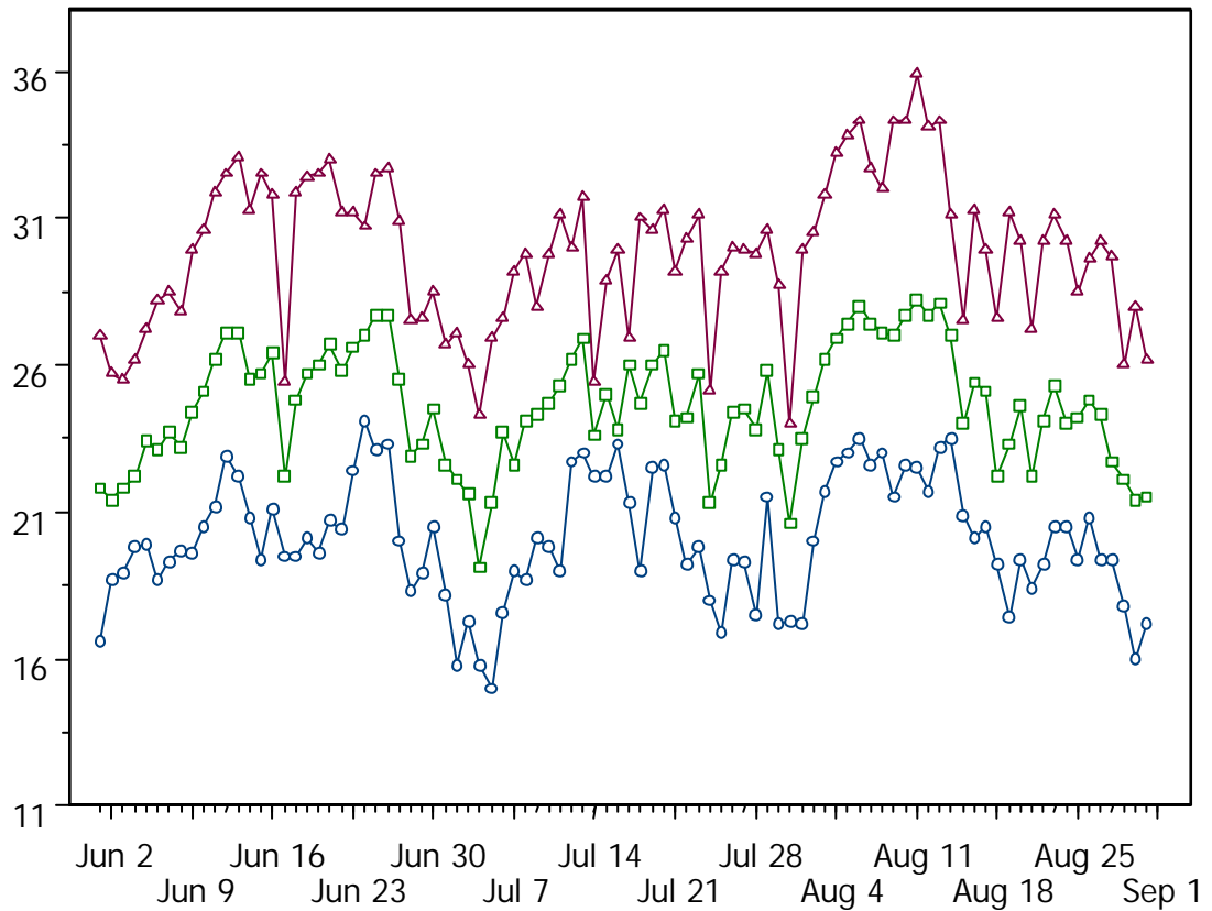
Grafico 3: Temperature giornaliere minime (in blu), medie (in verde) e massime (in rosso) osservate a Lugano tra il 1° giugno e il 31 agosto 2003. (Fonte: MétéoSuisse).
