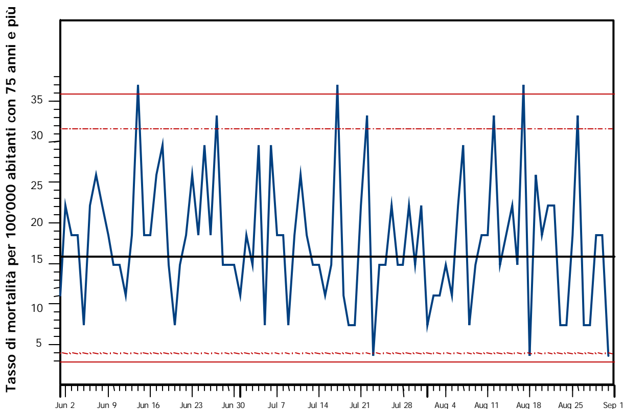
Grafico 12: Mortalità giornaliera per 100'000 abitanti con 75 anni e più osservata in Ticino nei mesi di giugno, luglio e agosto 2003. La mediana (linea nera), i quantili al 5% e 95% (linee tratteggiate rosse) e i quantili all'1% e 99% (linee continue rosse) sono stati definiti in base ai dati disponibili dal 2000 al 2002.
