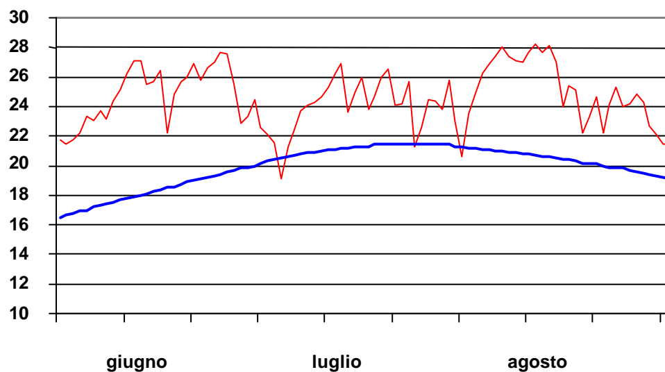
Grafico 2: Temperature medie giornaliere a Lugano (in rosso) e media plurienale (in blu). (Fonte: MeteoSvizzera).
